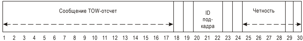
Рис. В-4. Формат слова NOW
