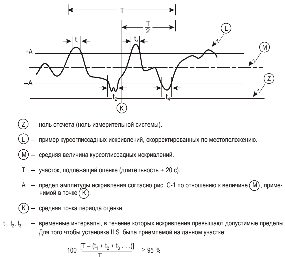
Рис. С-2. Оценка амплитуды курсоглиссадных искривлений
