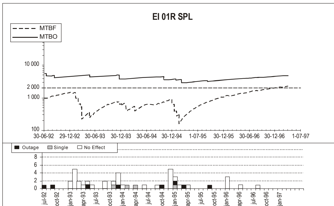
Рис. G-35B. Пример зарегистрированных данных о выходах из строя угломестного оборудования MLS
