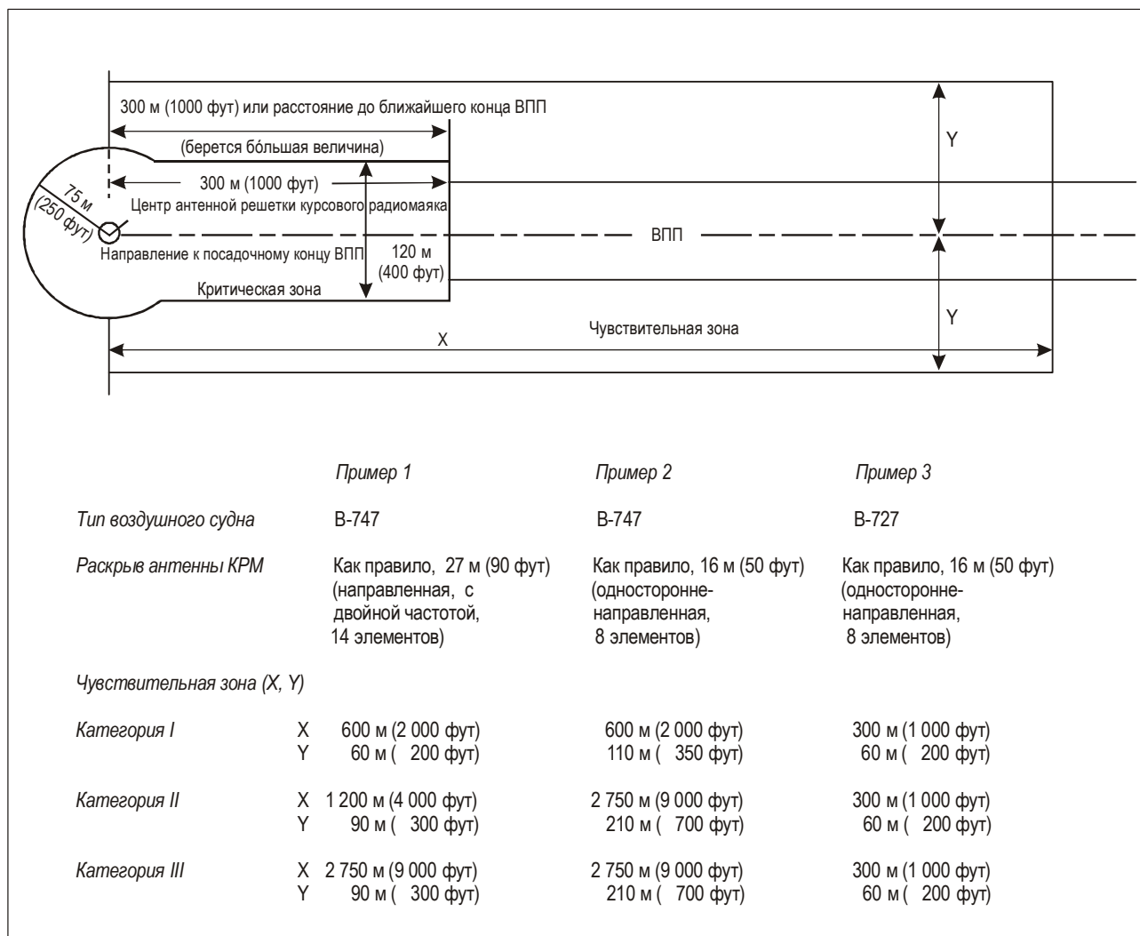
Рис. С-3А. Типовые изменения размеров критической и чувствительной зон КРМ для ВПП длиной 3000 м (10 000 футов)
