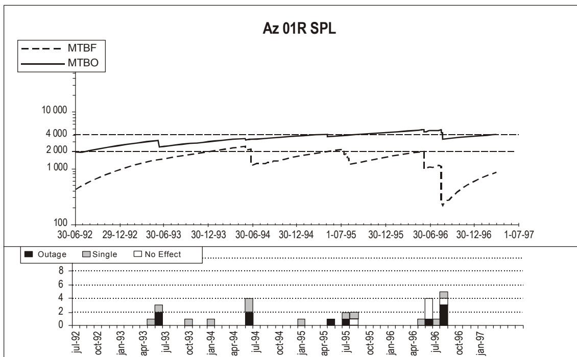
Рис. G-35A. Пример зарегистрированных данных о выходах из строя азимутального оборудования MLS
