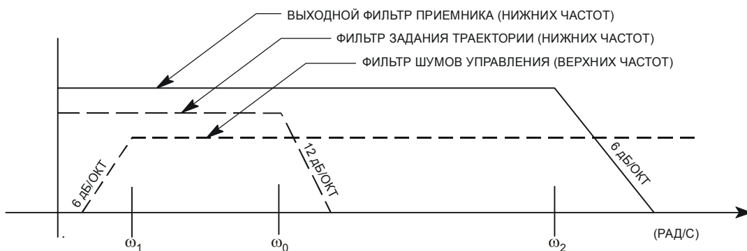
Рис. G-11. Конфигурации фильтра и частоты среза
