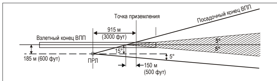
Рис. С-17. Минимальная удаленность ПРЛ от точки приземления при смещении от оси ВПП на 185 м (600 футов), когда сканирование производится в пределах 5 и 15° по магнитному пеленгу воздушного судна (QDR) относительно ВПП
