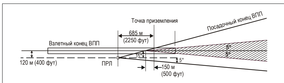
Рис. С-16. Минимальная удаленность ПРЛ от точки приземления при смещении от оси ВПП на 120 м (400 фут), когда сканирование производится в пределах 5 и 15^\circ по магнитному пеленгу воздушного судна (QDR) относительно ВПП
